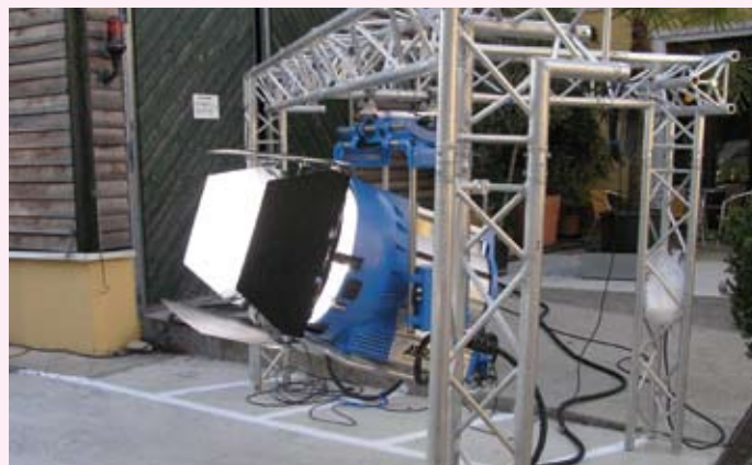
ARRI-MAX Scheinwerfer 12/18 kW
